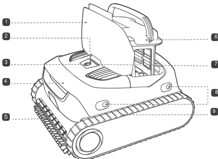
Роботизований очищувач басейнів (вид збоку)
