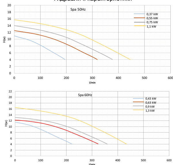
Гидравлич. характеристики
