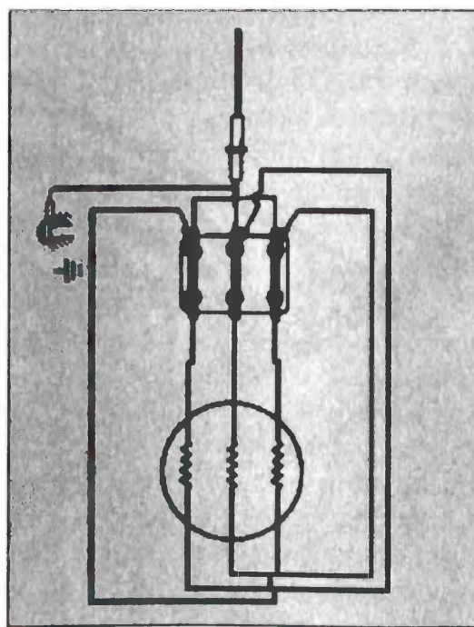
Соединение треугольником
