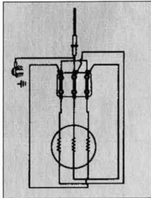
Соединение треугольником
