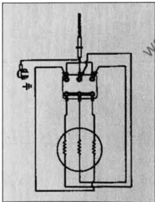
Соединение звездой
