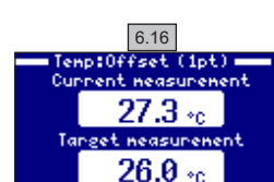
6.16 С помощью клавиш «плюс»/«минус» откорректируйте отображаемое датчиком значение так, чтобы оно совпадало с реальной температурой, затем нажмите ОК.
