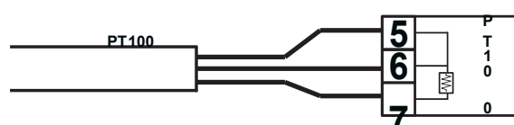
3-проводная схема подключения PT100
