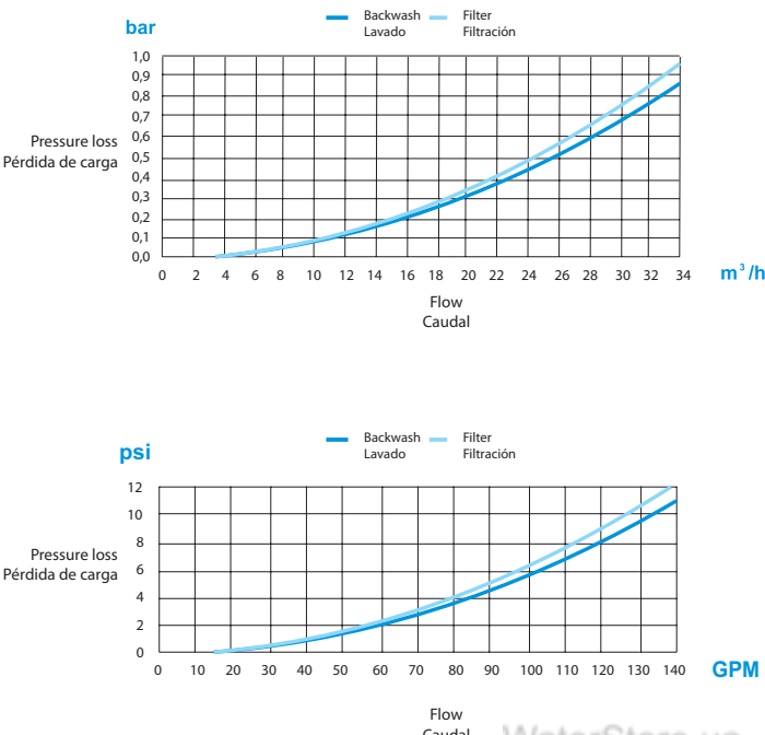
2" valve Válvula 2"
